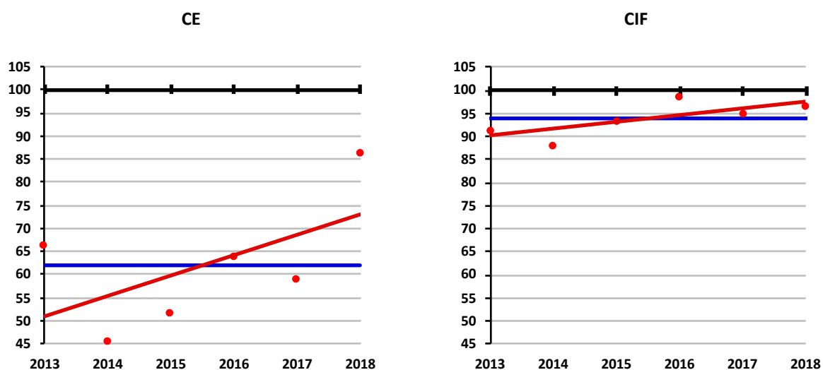
Figura 5.4.2.5.1 – Índices e declives no Agrupamento em Física e Química A, Ensino Secundário
