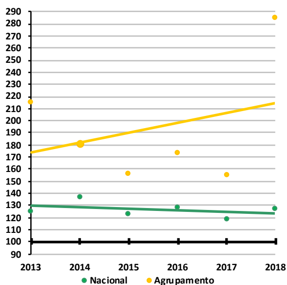
Figura 5.4.2.4.2 – Índices CIF e declives em Economia A, às escalas Nacional e do Agrupamento, Ensino Secundário
