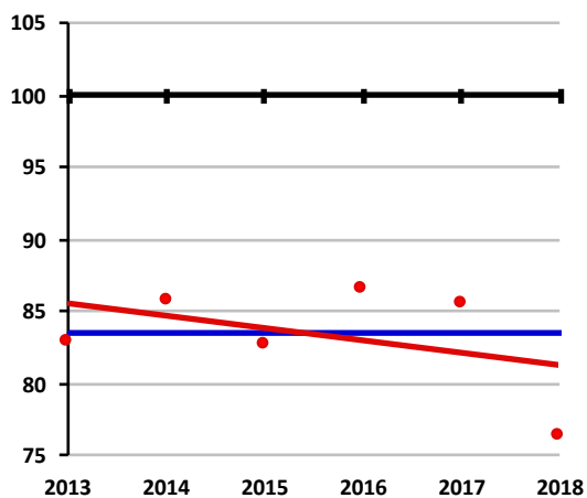
Figura 4.1.1 – Índices e Declives no Agrupamento segundo a Classificação de Exame (CE), 3º ciclo
