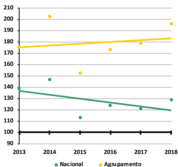
Figura 5.4.2.2.2 – Índices CIF e declives em Matemática A, às escalas Nacional e do Agrupamento, Ensino Secundário
