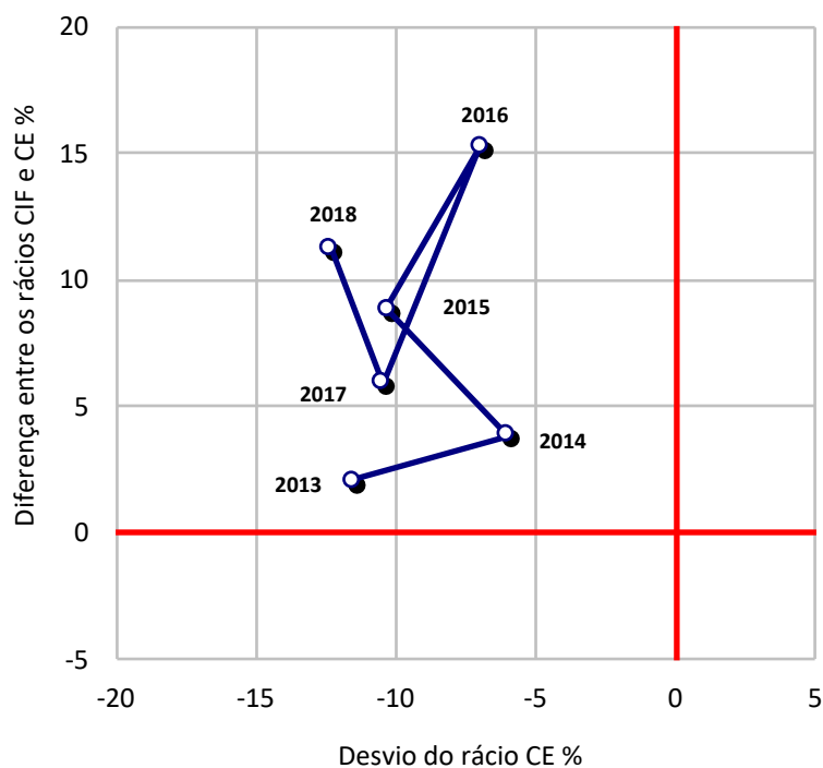
Figura 4.3.2.1 – Trajetória de relação entre a diferença rácio CIF - rácio CE (%) e o desvio do rácio CE (%) em Português, 3º ciclo - 2013 a 2018
