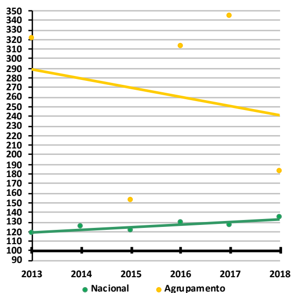
Figura 5.4.2.7.2 – Índices CIF e declives em Geometria Descritiva A, às escalas Nacional e do Agrupamento, Ensino Secundário
