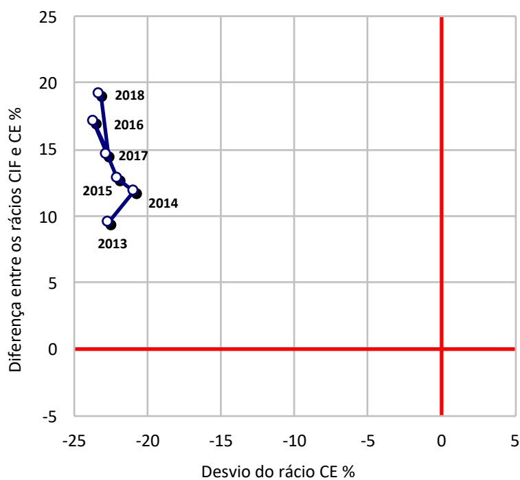
Figura 5.3.1 – Trajetória da relação entre a diferença rácio CIF-CE (%) e o desvio do rácio CE (%) no Ensino Secundário – 2013-2018
