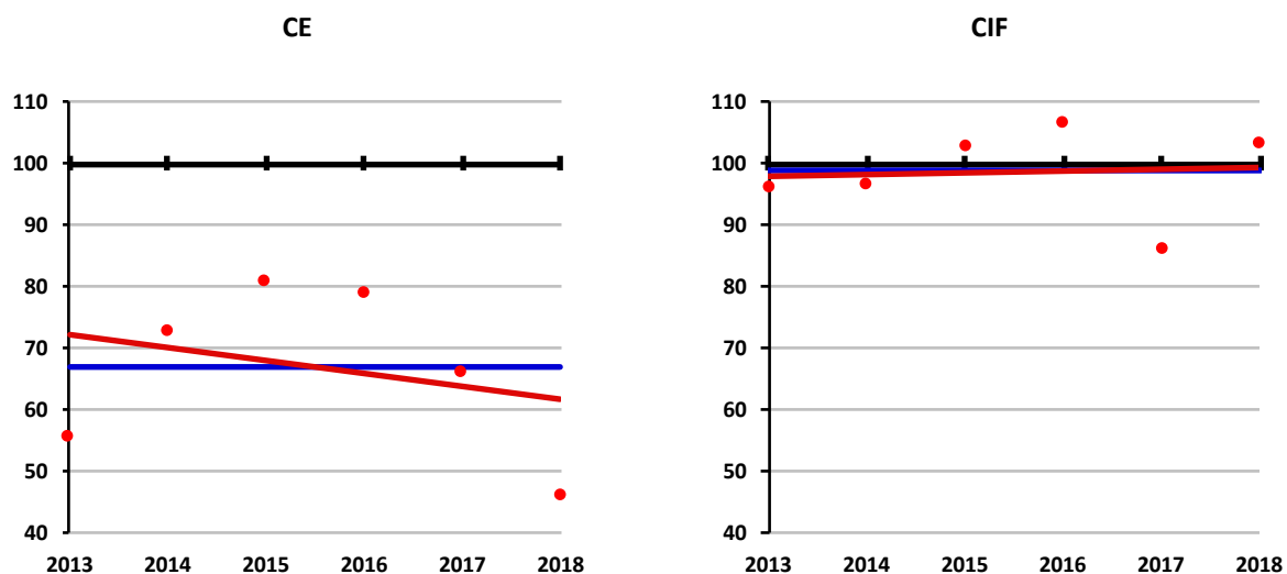
Figura 5.4.2.4.1 – Índices e declives no Agrupamento em Economia A, Ensino Secundário
