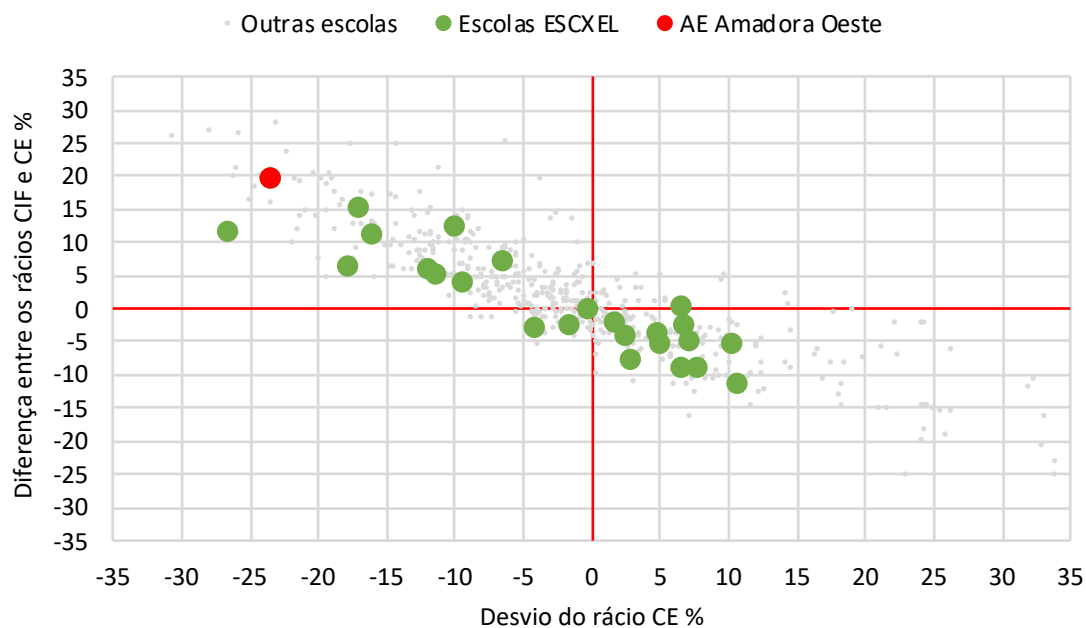
Figura 5.3.2 – Relação entre a diferença rácio CIF - rácio CE (%) e o desvio do rácio CE (%), Ensino Secundário – 2018
