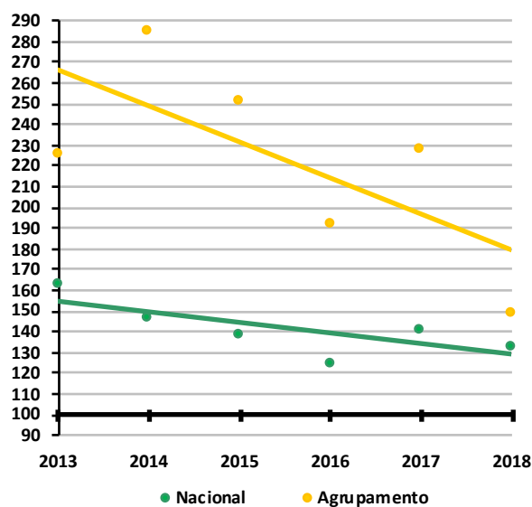
Figura 5.4.2.5.2 – Índices CIF e declives em Física e Química A, às escalas Nacional e do Agrupamento, Ensino Secundário
